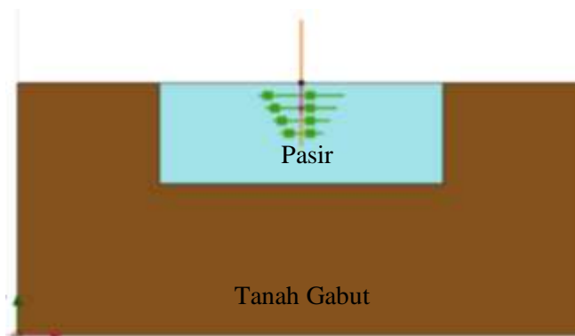
Gambar 4. Pemodelan Fondasi Kacapuri yang telah Dimodifikasi Menggunakan Empat Strip Plat Kayu Ulin Sumber: Hasil Analisis (2025)
