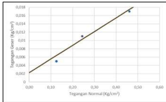
Gambar 3. Grafik Hubungan Tegangan Normal dan Tegangan Geser Sumber: Hasil Analisis (2025)
